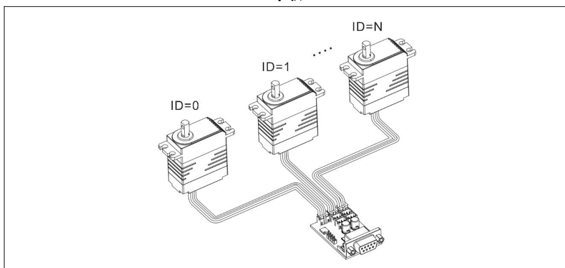
并联
